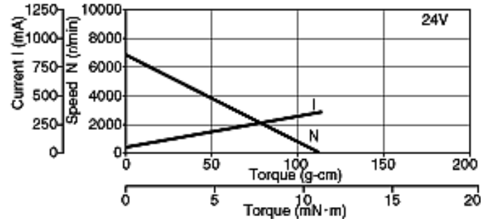
EN22 24V type
