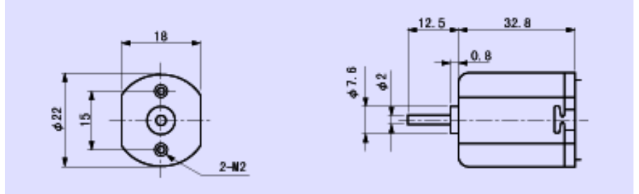
EN22 24V type
