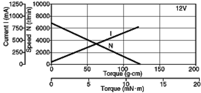
EN22 12V type
